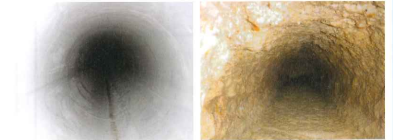
▲正常な下水道本管
