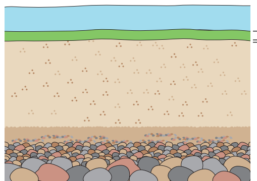
微生物膜
