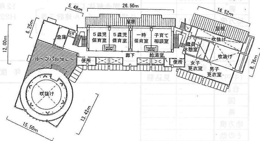
2階平面図
