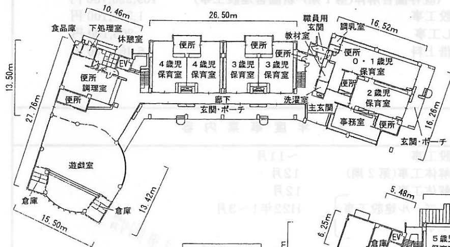
1階平面図
