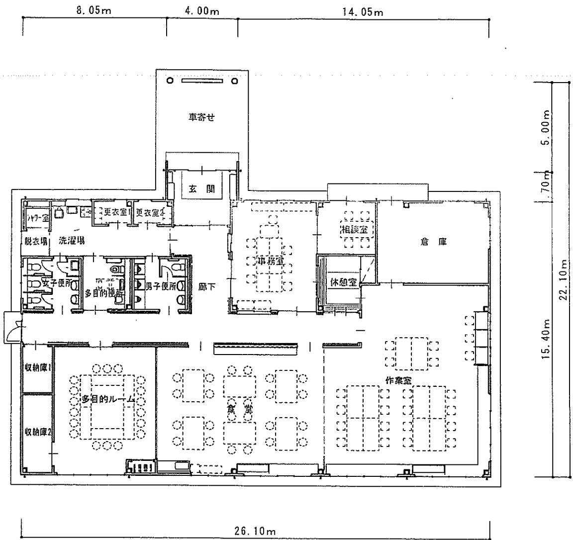
平面図
