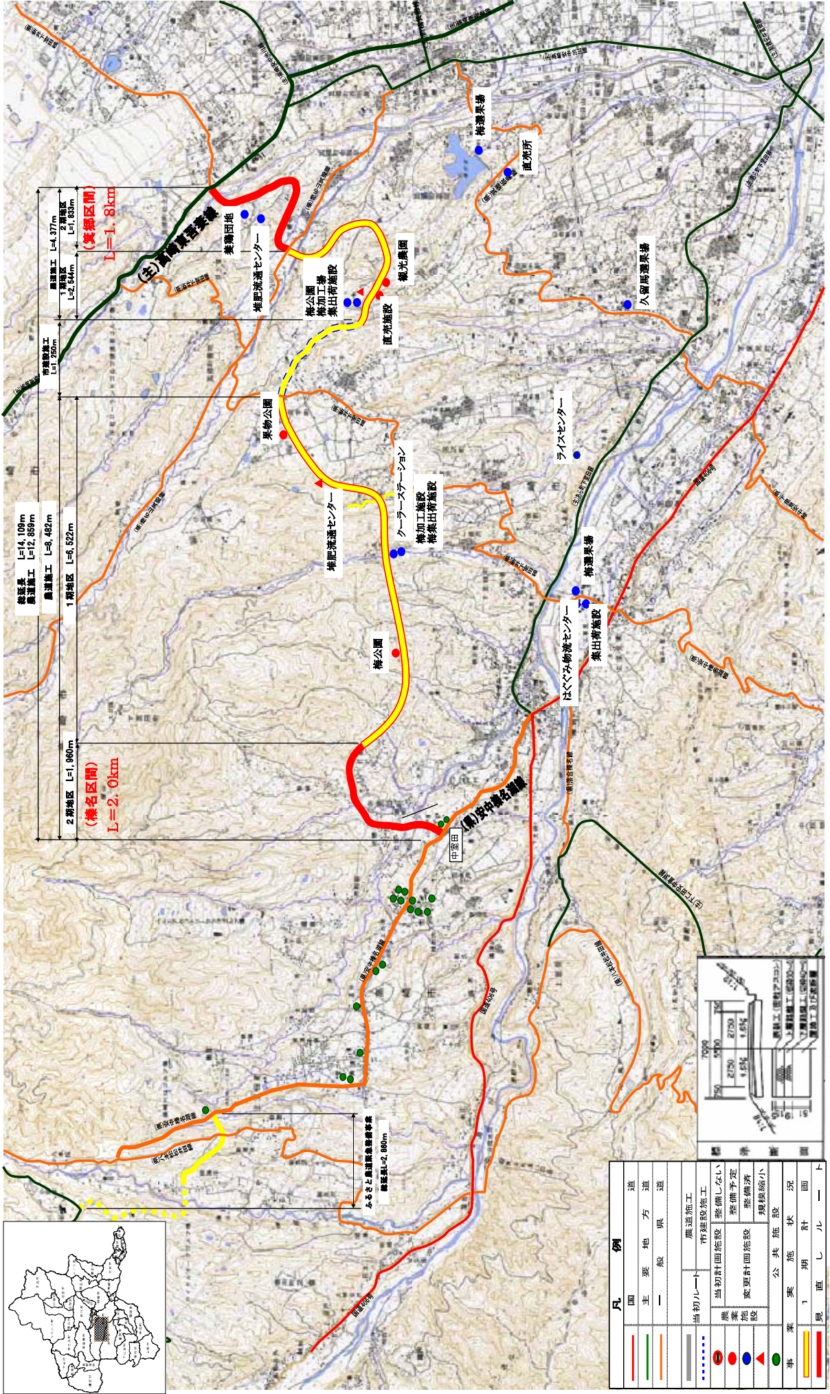
県営広域営農団地農道整備事業 榛名南麓2期地区 計画一般図
