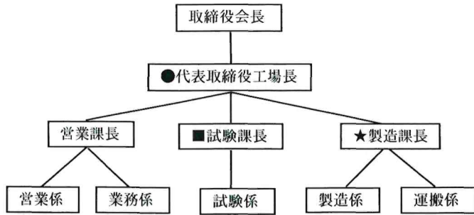
(管理体制図)
