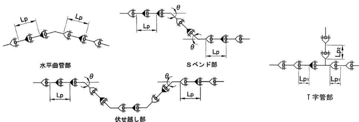
曲管部および T 字管部の一体化長さ（呼び径 75～300） 単位：m
