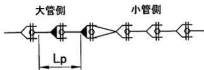
片落管部の一体化長さ
