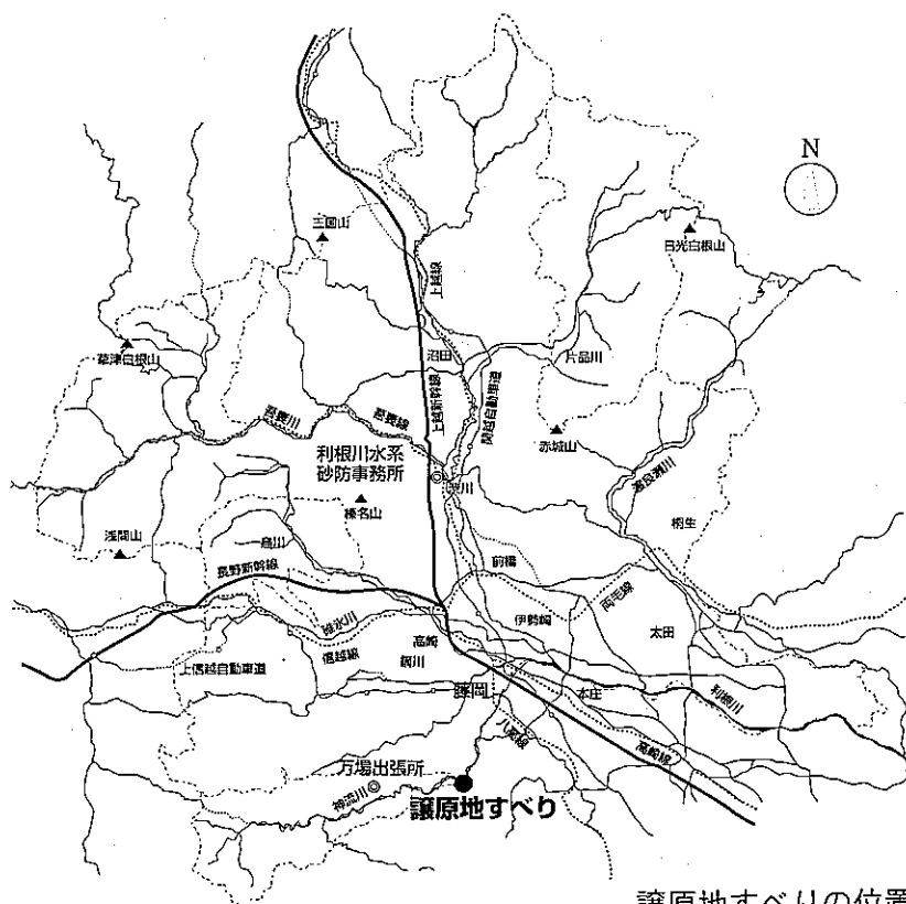
譲原地すべりの位置
