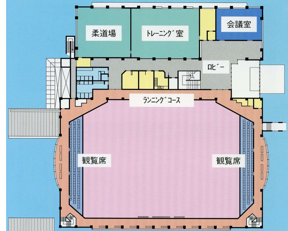
2 階平面図
