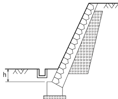
図 3-20 U字溝に接する場合の根入れ
