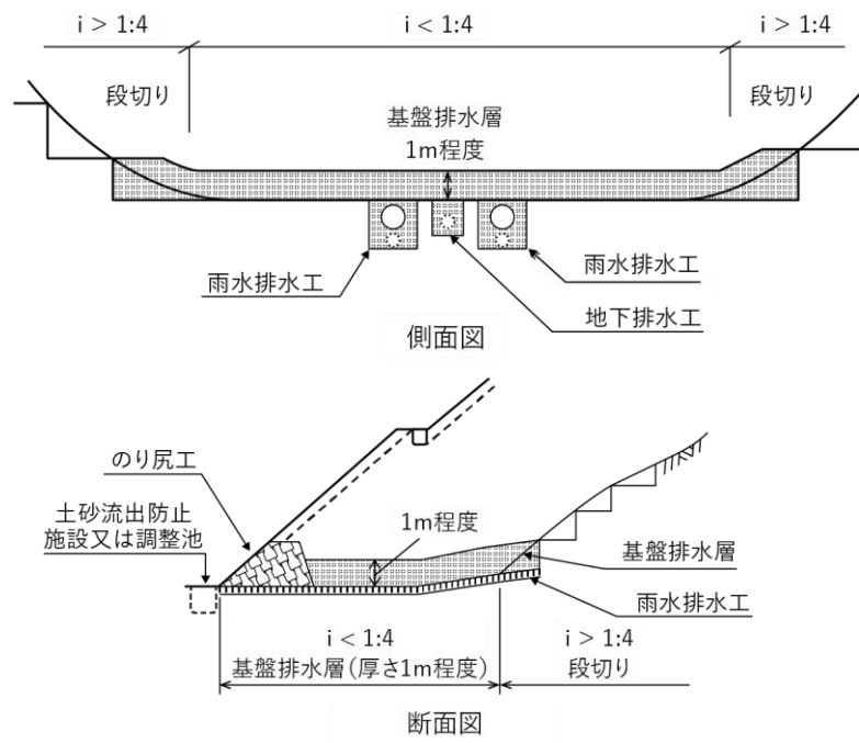
図 3-48 基盤排水層
