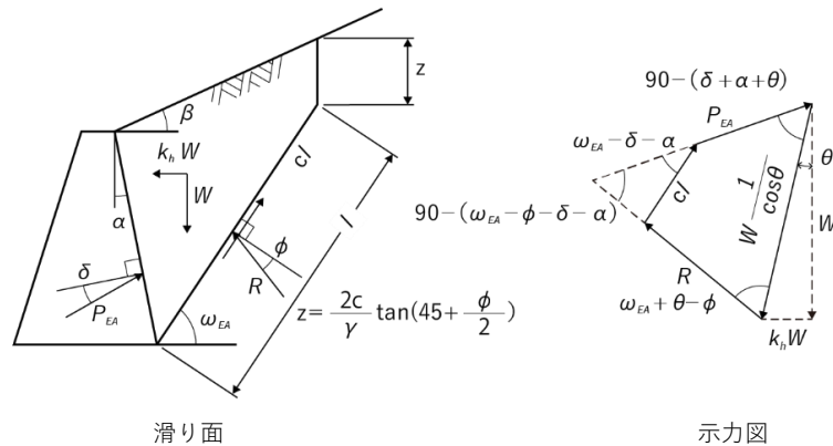
図 3-33 裏込め土が粘着力を有する場合の地震時主働土圧
