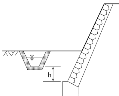
図 3-19 水路に近接する場合の根入れ
