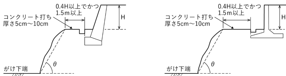
図 3-16 斜面上に設置する擁壁の構造
