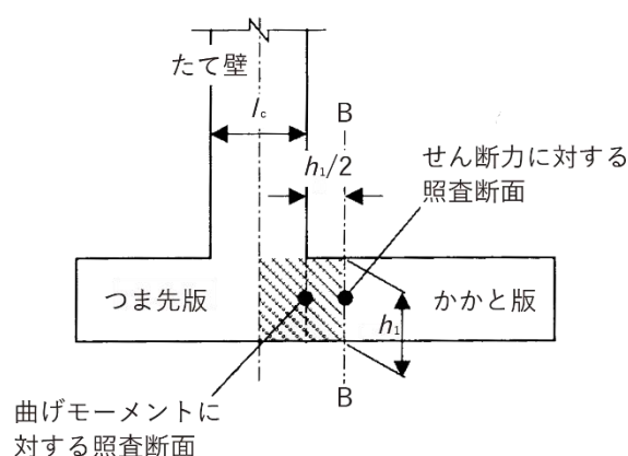
図 3-42 かかと版のせん断力を照査する断面
