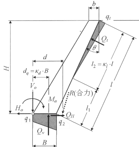
図 3-37 地盤反力係数法（簡便法）
