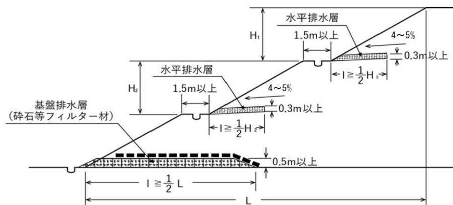
図 3-49 水平排水層
