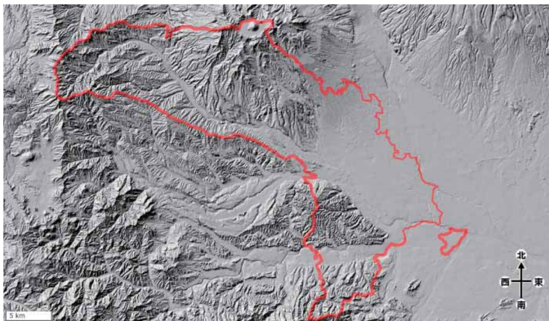
図1-3 高崎市の地形（国土地理院陰影起伏図に加筆）
