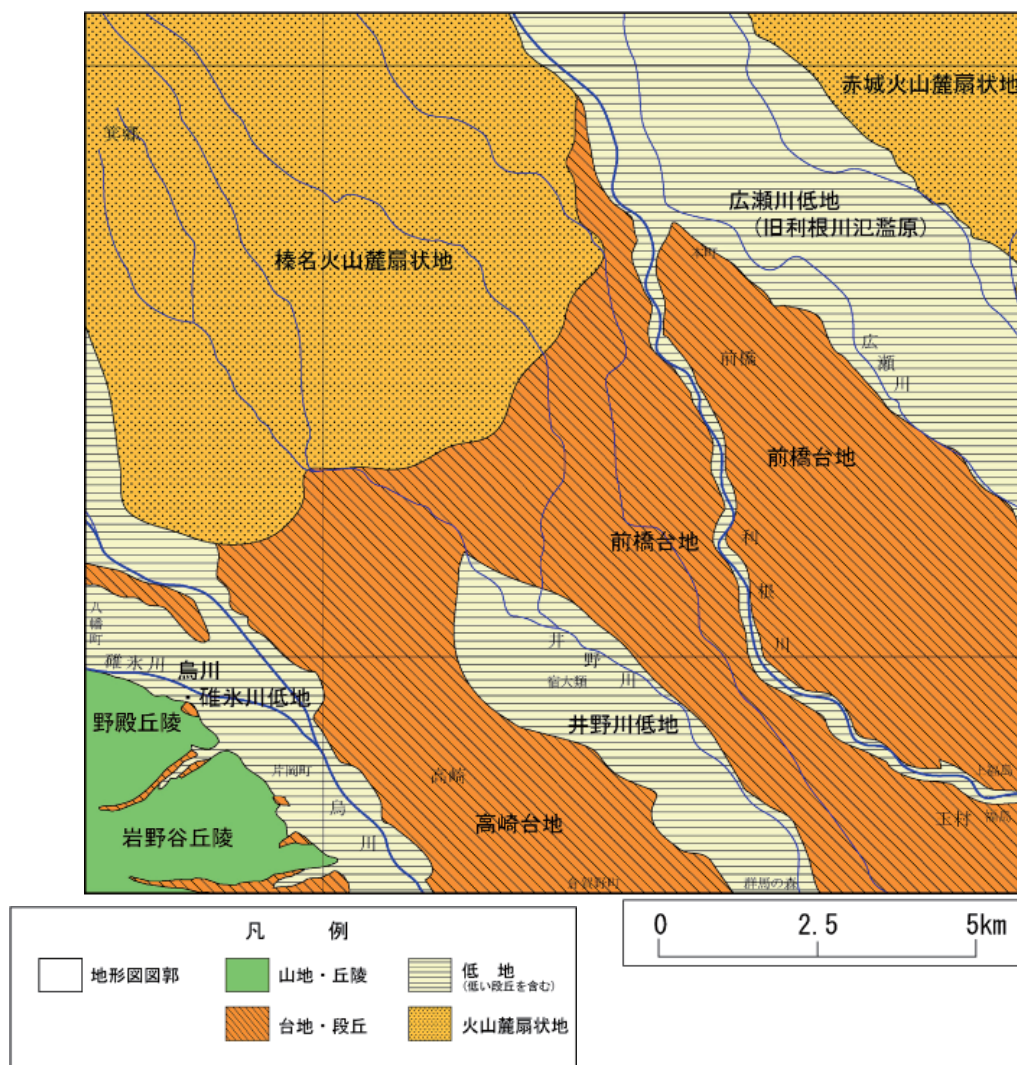
図1-4 地形地域区分図 ( 国土地理院土地条件調査解説書「前橋及び高崎地区」の図に加筆)
