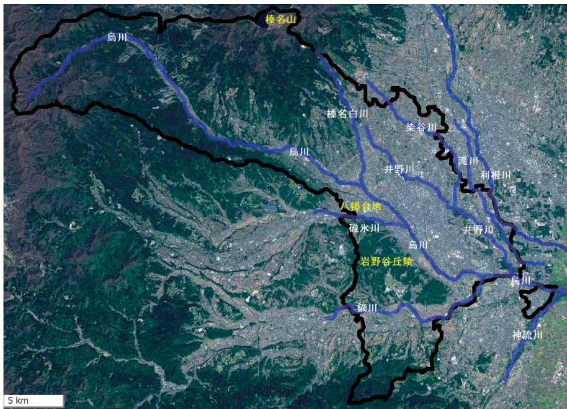
図1—8 主な山や河川の位置（国土地理院地図 GSI Maps に加筆）
