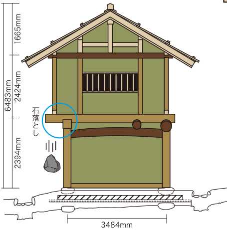
側面図及び基礎断面図
