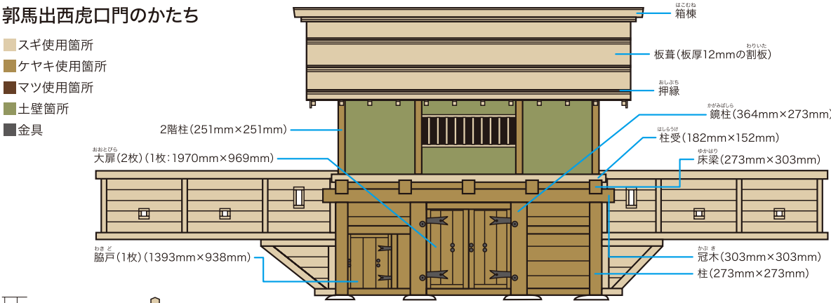
立面図
