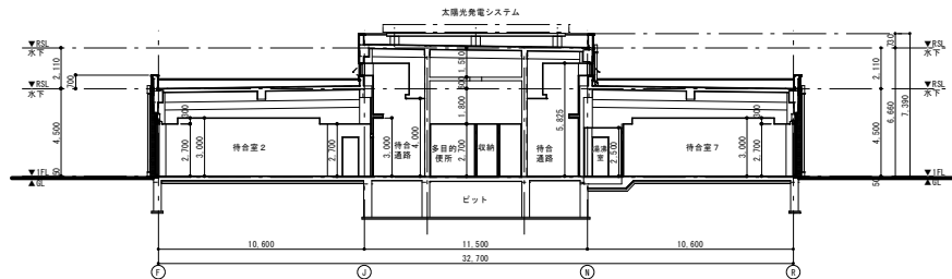
待合棟 F-R 断面図
