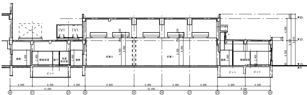
式場棟 20-30 断面図
