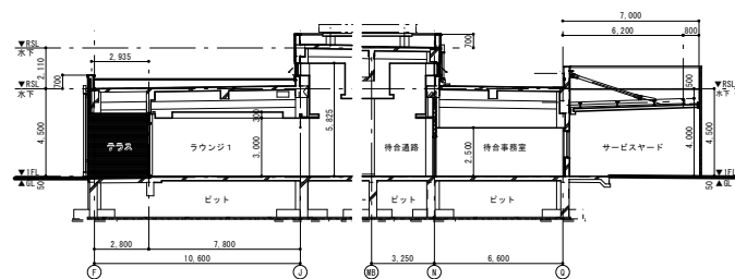
待合棟 F-0 断面図
