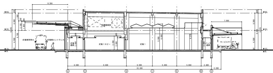
式場棟 A-0 断面図
