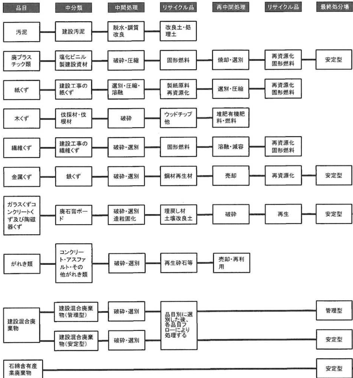
(第1面) ④ 産業廃棄物の一連の処理の工程
