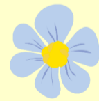
観劇
