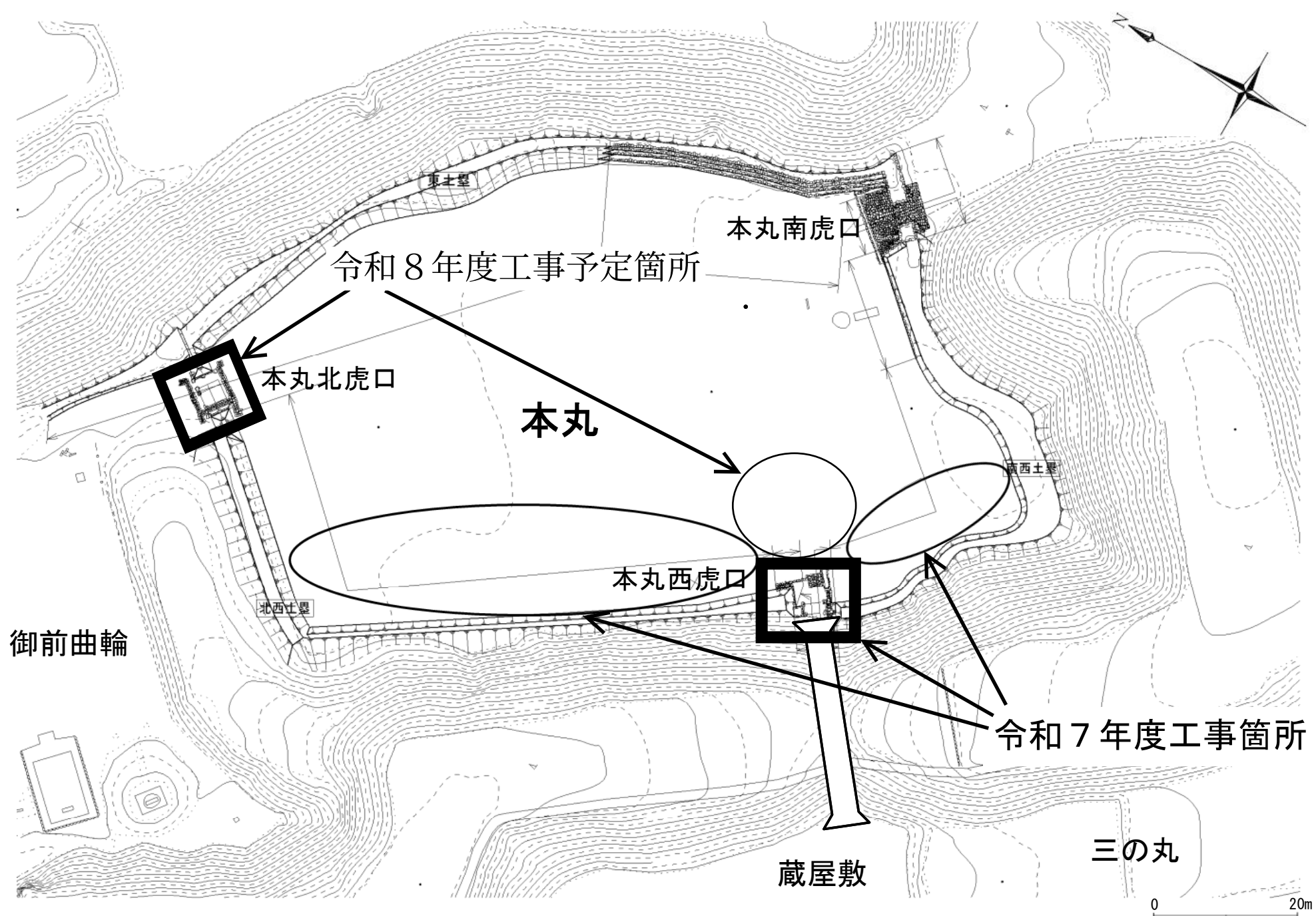
箕輪城跡本丸地区整備工事位置図
